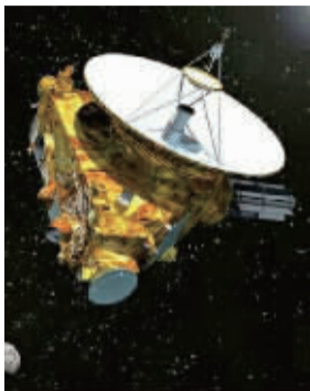
“新视野”号探测器
