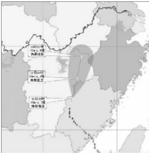
“莫兰蒂”路径概率预报 (15日19时~16日07时)
