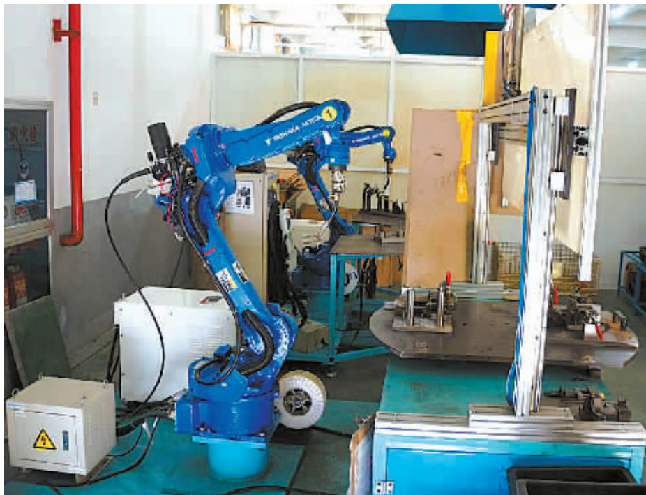
宁波福士汽车部件有限公司进行机器人改造后由手工焊接改为机器人自动焊接,既降低了生产成本又提高了生产效率。(冯璋 摄)
