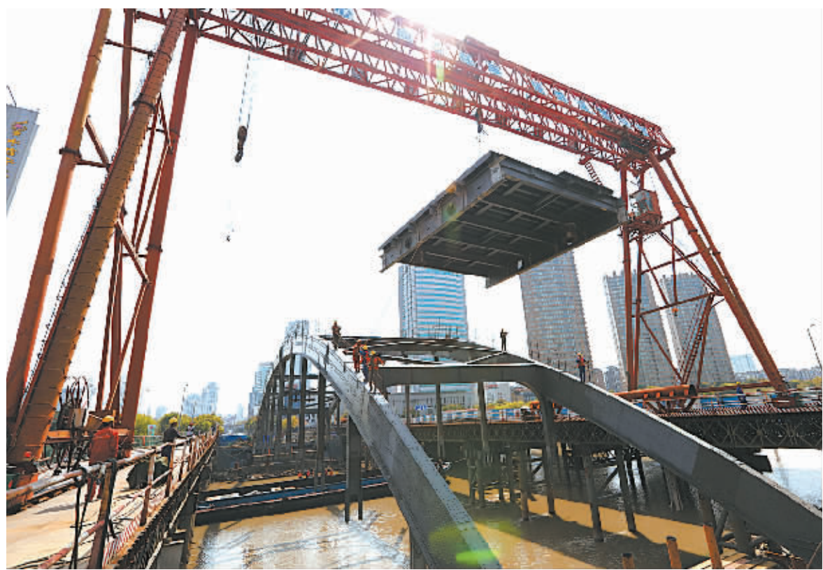
图为首批桥面板运达灵桥大修现场。(董娜 周骏 摄)
