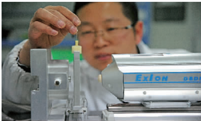
在宁波华仪宁创智能科技有限公司实验室,科研人员正在对“DBDI-100型介电阻挡放电质谱离子源”进行校准。(徐能 虞文未 摄)
