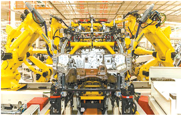
吉利汽车春晓基地焊装车间
