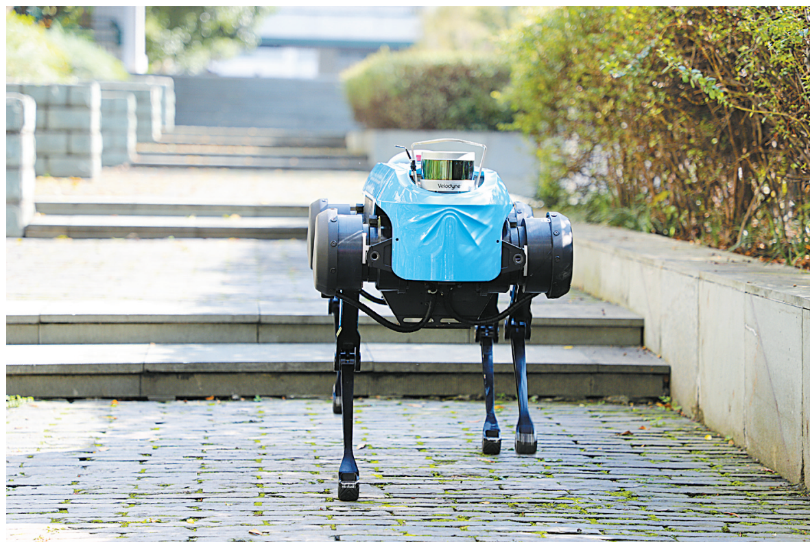
“绝影”四足机器人在有台阶的环境中稳定行走(11月24日摄)。
