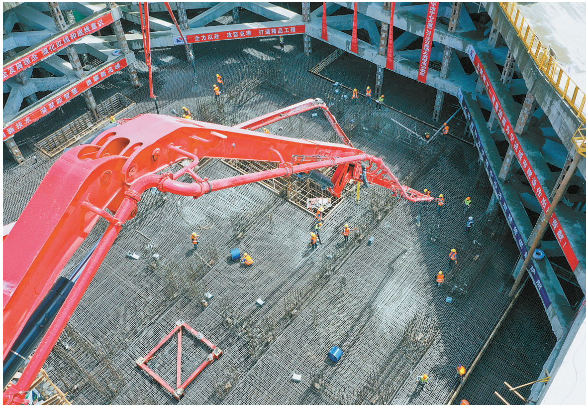
宁波中心大厦基础底板浇筑现场。
