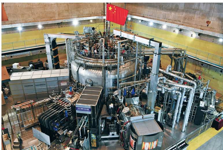
这是有“人造太阳”之称的全超导托卡马克核聚变大科学装置 EAST。（新华社发）
