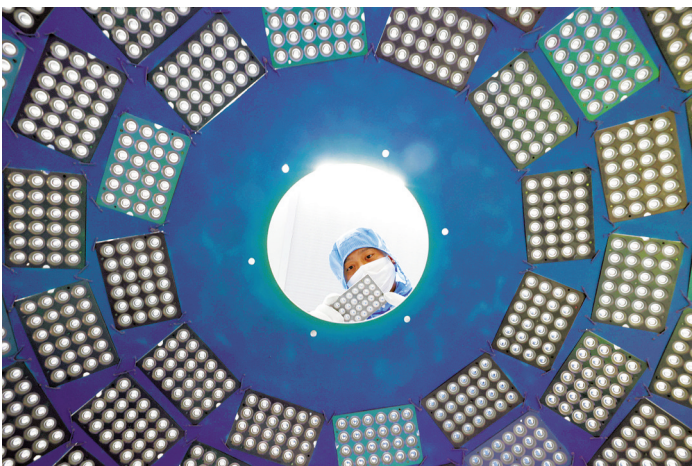
镜头镀膜是决定镜片透光性能的关键一步,图为工作人员正在进行镀膜前检查。
