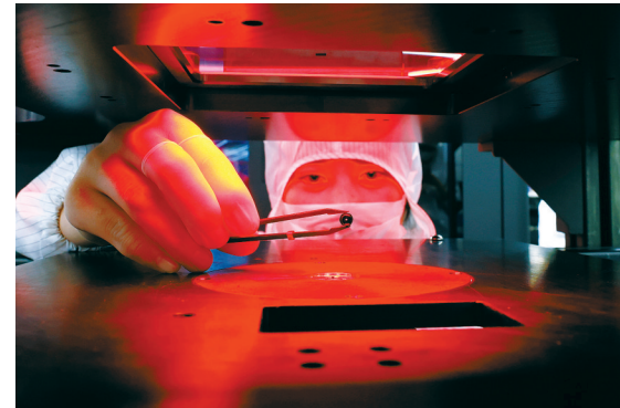
工作人员正在用光学功能检查仪检测镜头。
