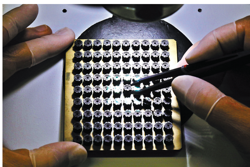
工作人员正在对镜头进行检测。
