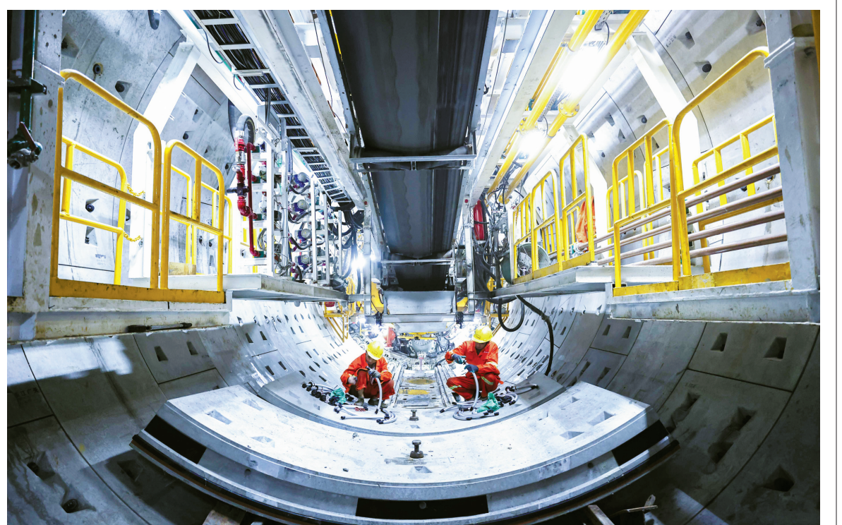
施工人员在盾构机内进行管片拼装作业。
