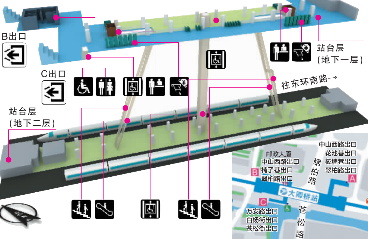
车站站层图
