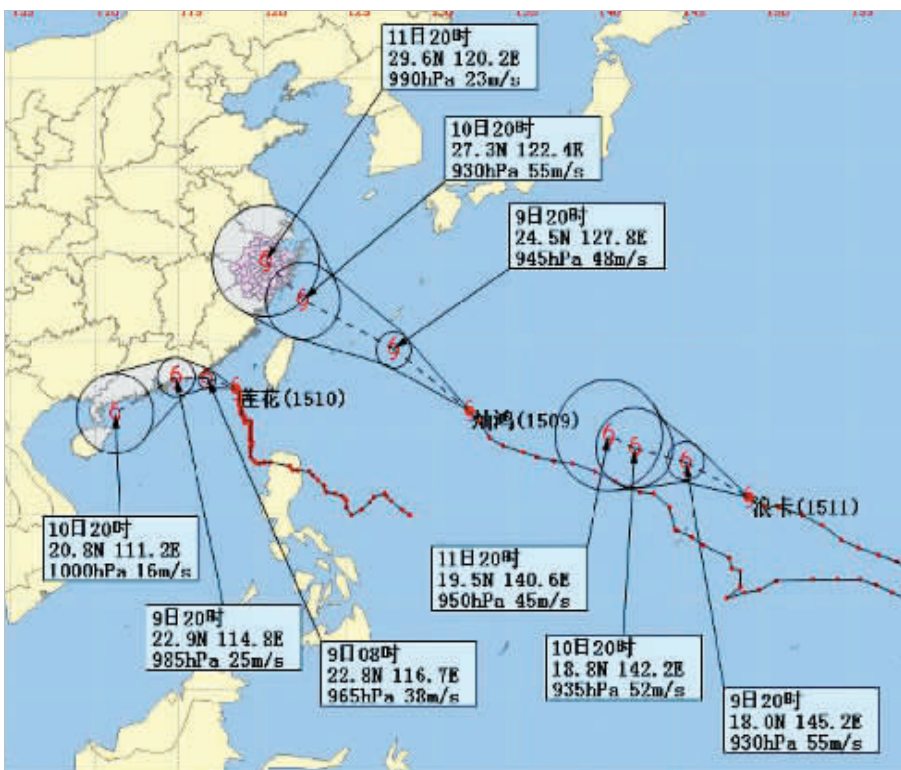
“灿鸿”、“莲花”和“浪卡”未来72小时路径概率预报图(昨天20时发布)。图片来源:浙江天气网
