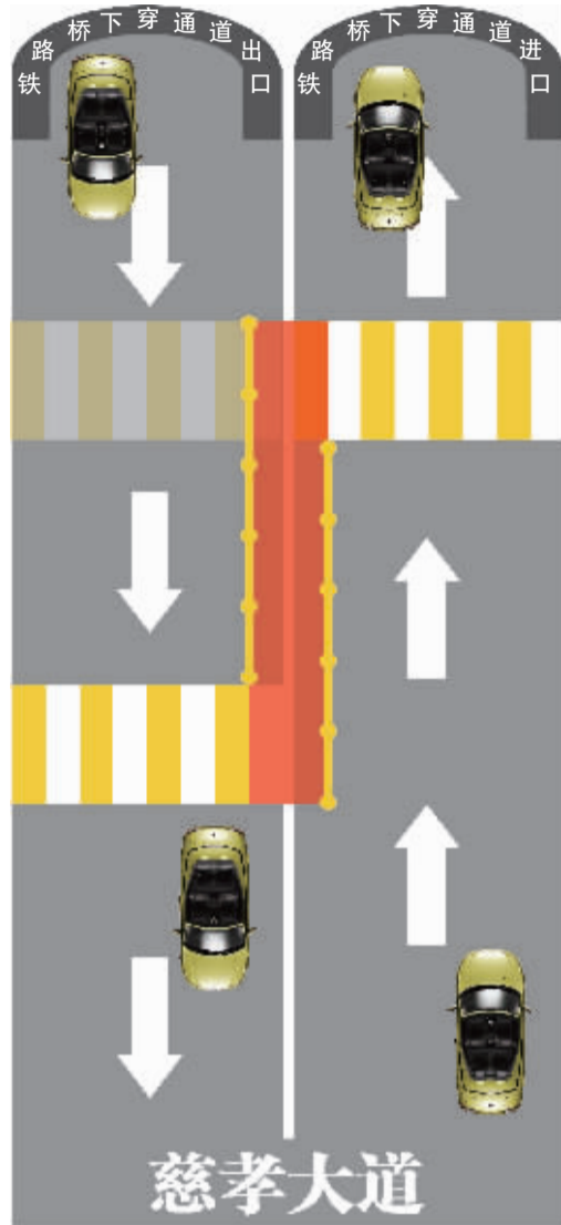
“错位过街”设施示意图，图中红色区域为连接两侧斑马线的、用隔离栏拦出来的通道。 严勇杰 制图
