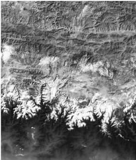
高分四号卫星珠穆朗玛峰影像
