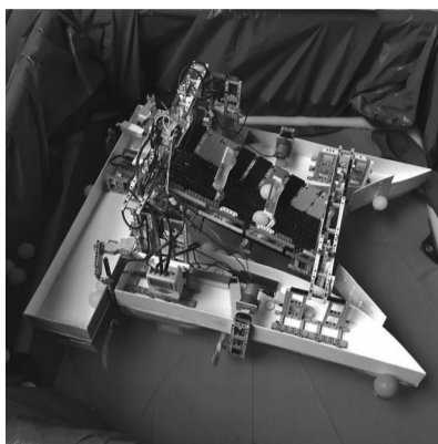
对接好的运输船和收集船。
