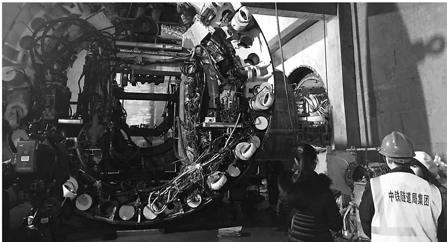
宁波轨道交通4号线盾构施工现场。记者 王元卓摄
