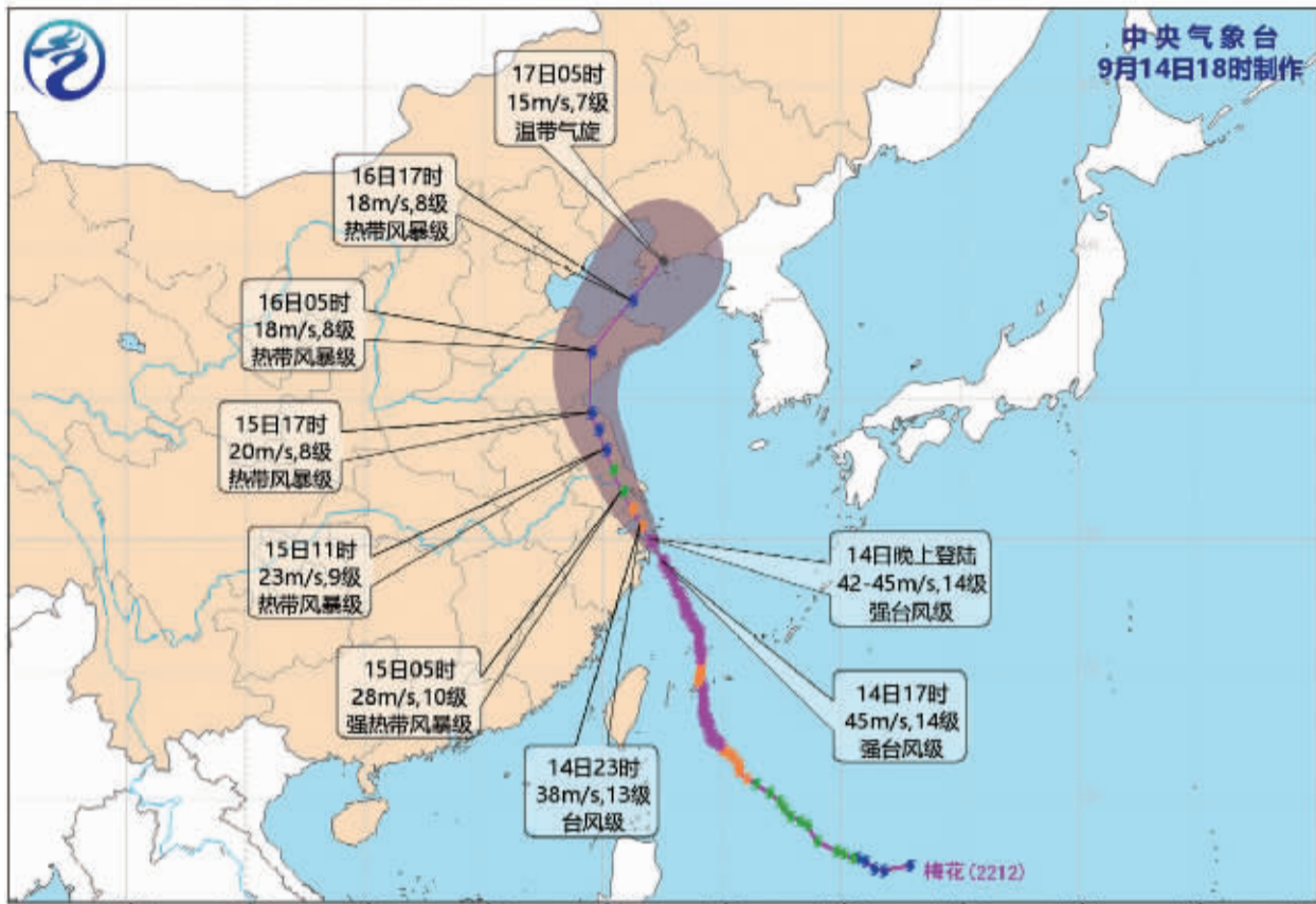
今年第12号台风“梅花”未来60小时路径概率预报图 2022年9月14日17时—17日05时(北京时间)
