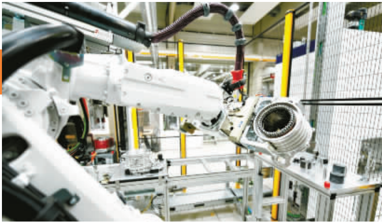
戴姆勒奔驰电驱转子定子装配线。
