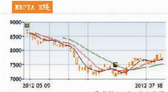
甬商所PTA的K线走势图
