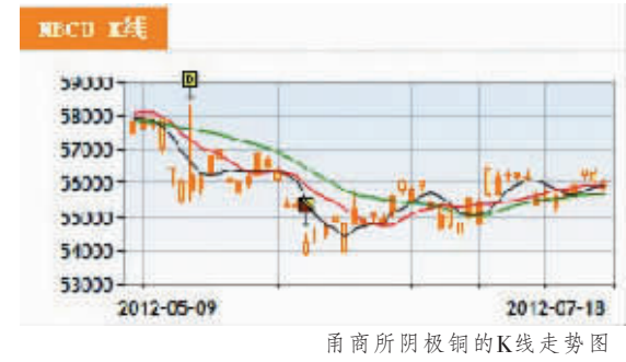
甬商所阴极铜的K线走势图
