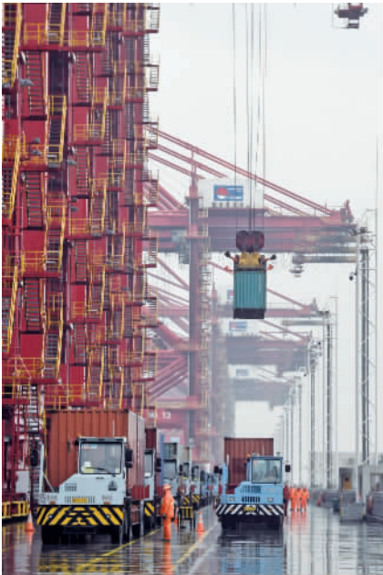
宁波舟山港梅山岛国际集装箱码头,工人使用桥吊为货轮装卸集装箱。
